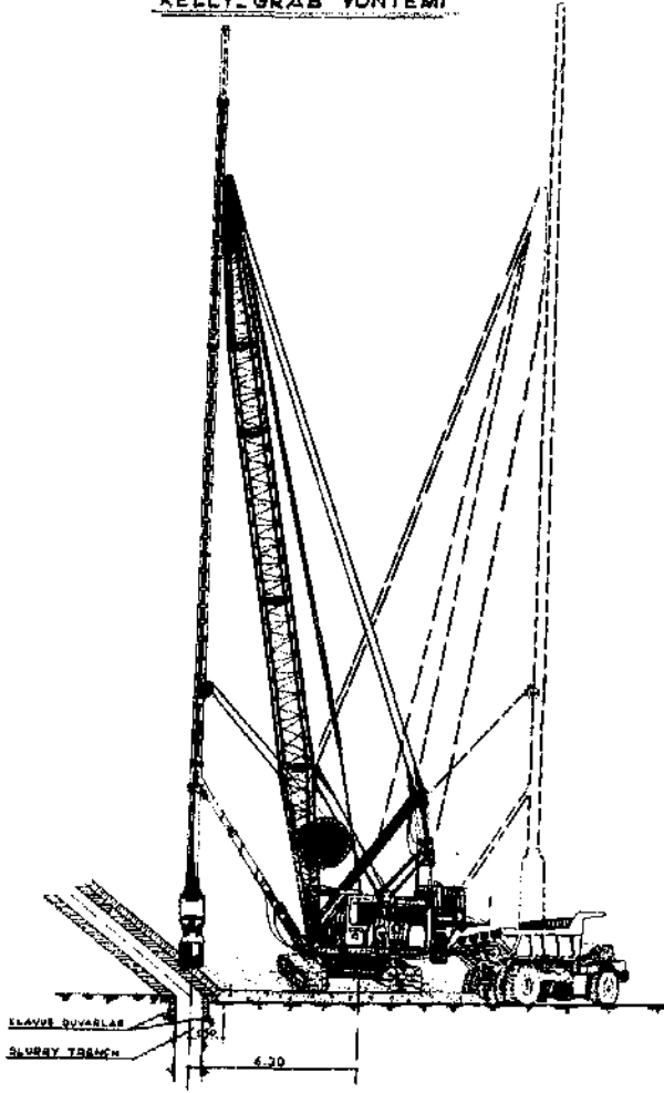
Şekil 3: Slurry - Trench için Kelly-Grab yöntemi.
