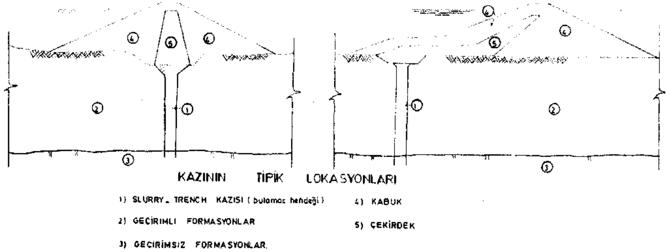
Şekil 2: Kazının tipik lokasyonları,
