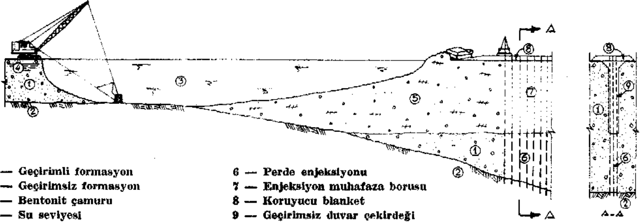
Şekil 11 Perde enjeksiyonu ile geçirimsizlik duvarı çekirdeği yapımı*
