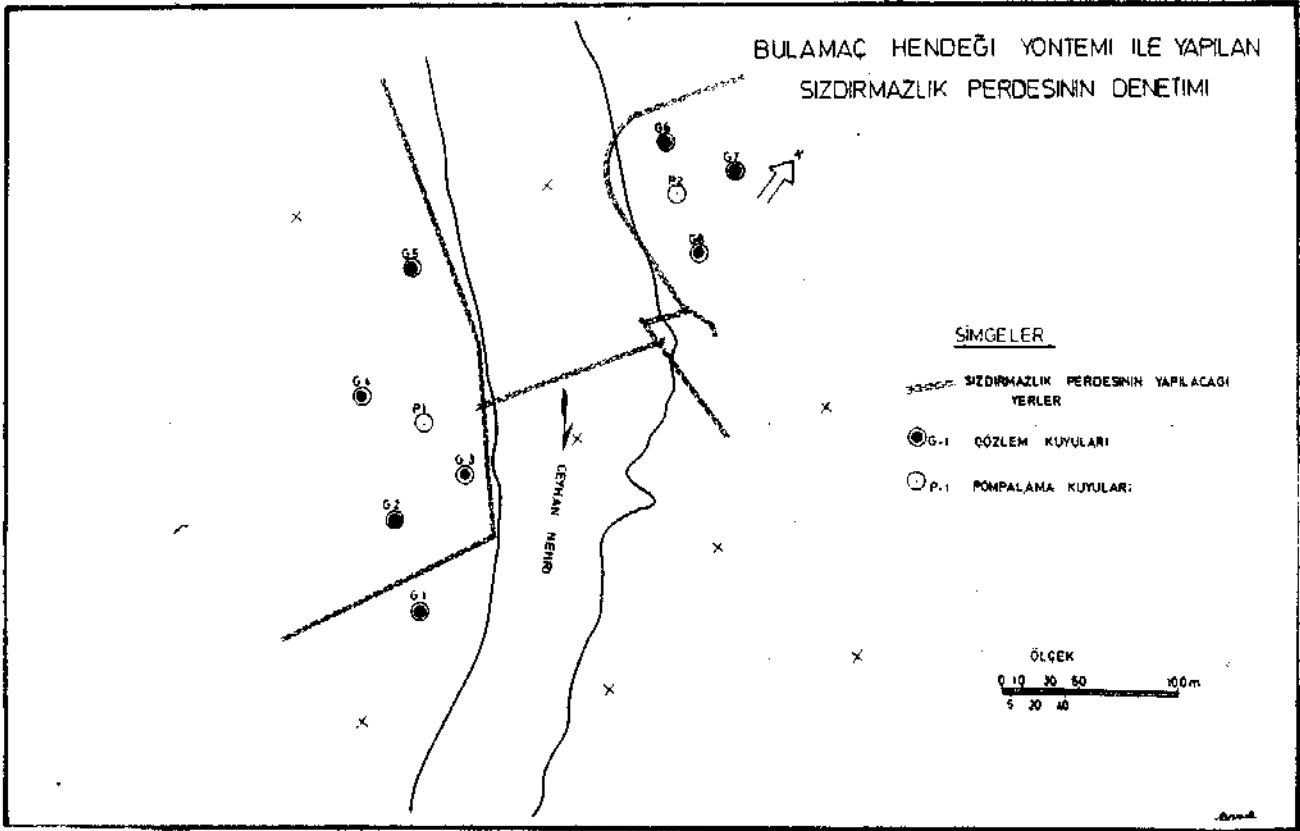
Şekil 6: Bulamaç hendeği yöntemi ile yapılan sızdırmazlık perdesinin denetimi.
